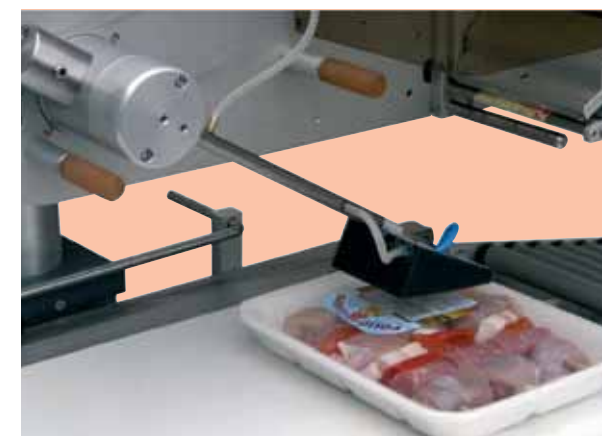
ETICHETTATURA CON APPLICATORE A BRACCETTO
